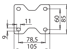
Priroba DIN: za kolesa Ø80 - Ø125
