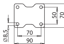
Priroba: za kolesa Ø100, Ø125
