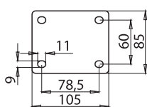
Priroba DIN: za kolesa Ø80 - Ø125 DIN top plate: for castors Ø80 - Ø125
